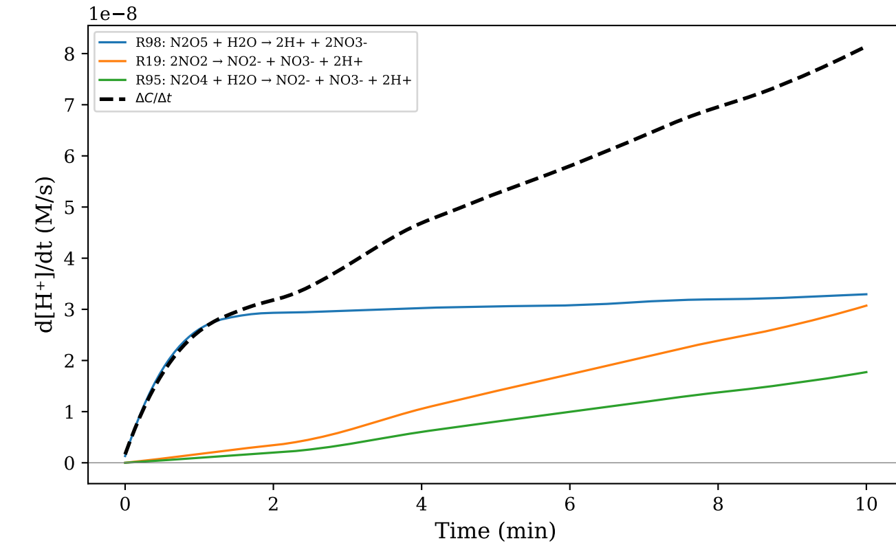
(d) H + [final=30.45 μM]
